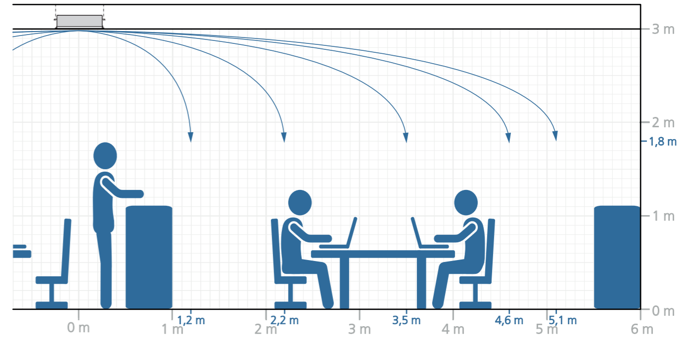
KaDeck zweiseitiger Luftauslass, 16/18/27 °C
