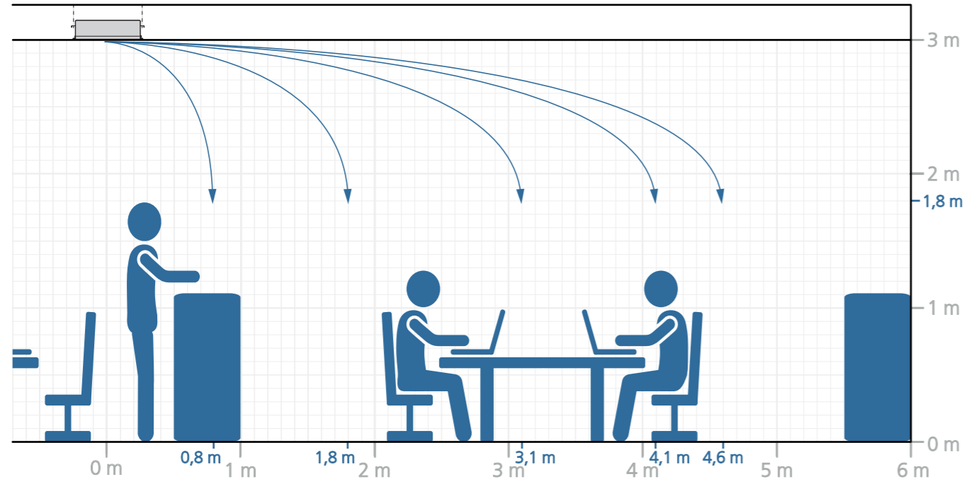
KaDeck einseitiger Luftauslass, 7/12/27 °C
