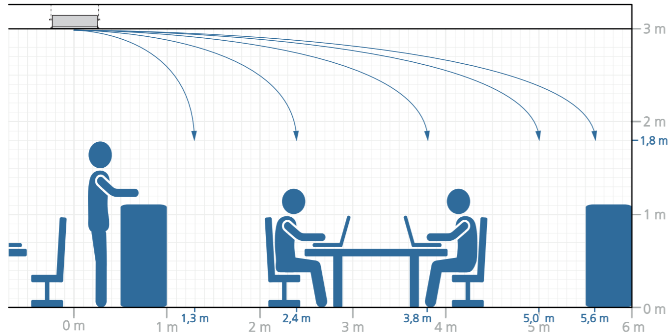
KaDeck einseitiger Luftauslass, 16/18/27 °C
